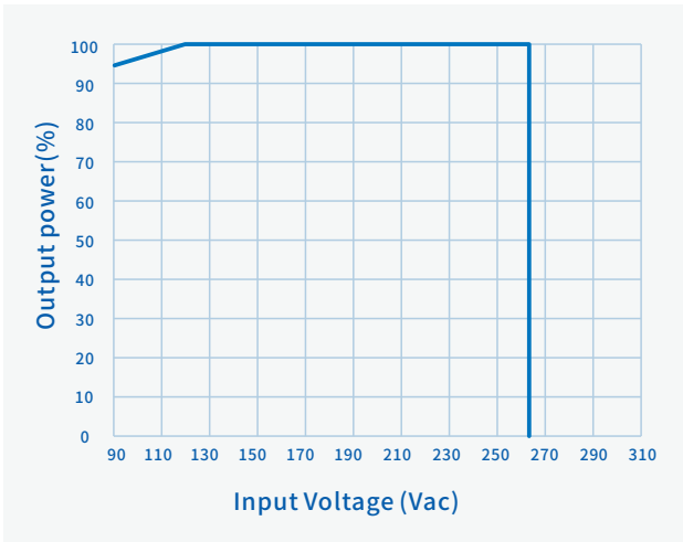
输出功率Vs.输入电压(Ta:25℃)
